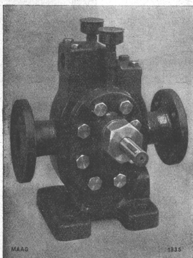
MAAG-ZAHNRADPUMPE mit Heizmantel zur Förderung von Schwefel- Teer bei 120° C.
