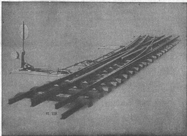
Zahnstangenweiche Jungfraubahn.
