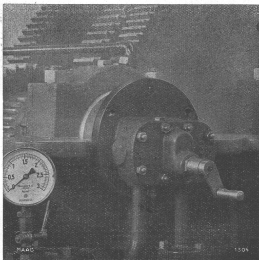
MAAG-ZAHNRAD-SCHMIERPUMPE für Turbogetriebe, mit Handantrieb, zur Erzeugung des Öl- druckes während des Anlaufens der Maschine.
