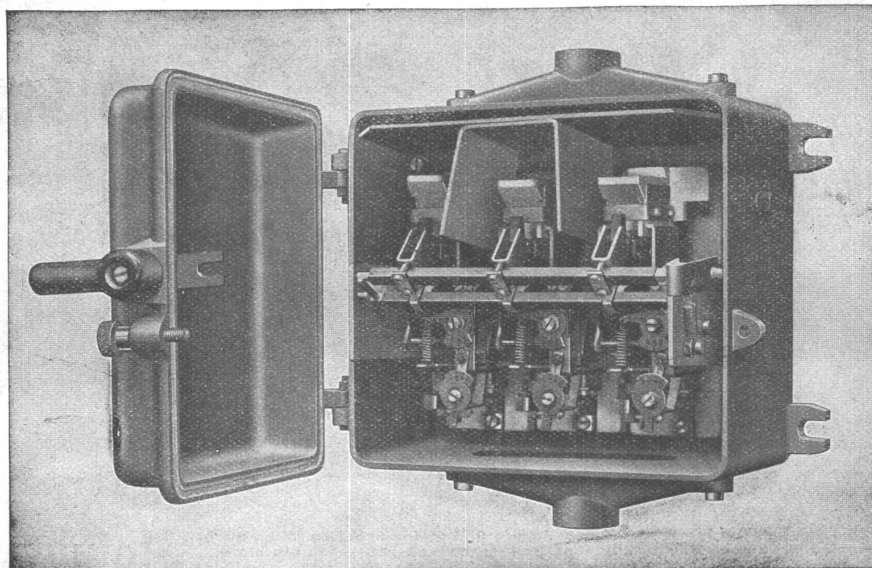
Schutzschalter für Drehstrom-Motore bis 500 Volt, 25 Amp.
