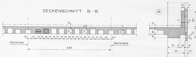
Abb. 12. Deckenschnitt B-B (in Abb. 13) und Fassadenträgerschnitt A (in Abb. 14). 1 : 80.
