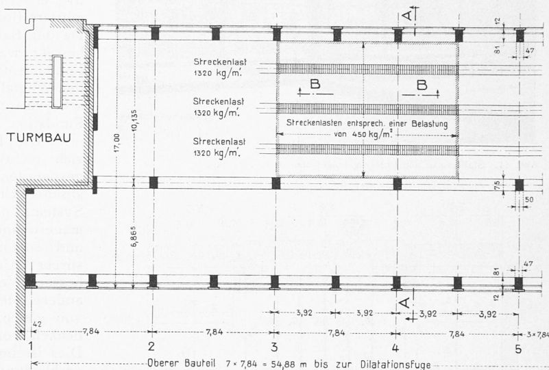
Abb. 13. Oberer Bauteil, linke Hälfte. — Teilgrundriss vom 3. Stock, Masstab 1 : 300.
