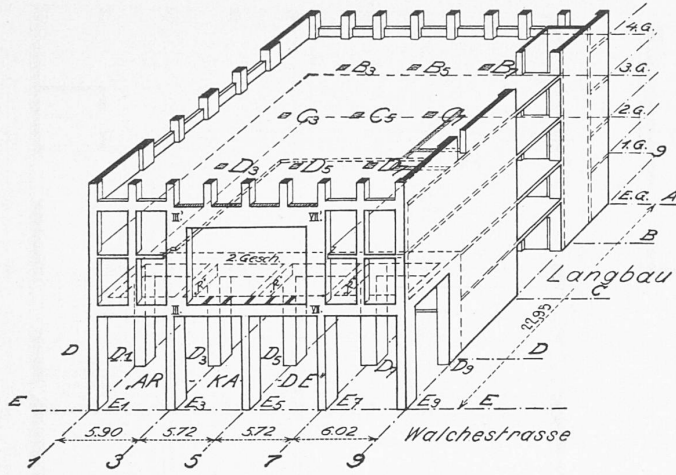
Abb. 7. Isometrie (1 : 500) der untern Geschosse des Turmbaus. Armierter Betonkonstruktion, soweit sie an der Aufnahme des Winddrucks auf die Fassaden beteiligt sind.
