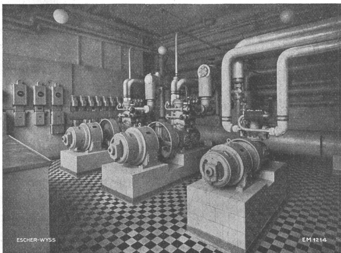
Vollautomatische „Frigotrop“-Kühlanlage der Gross-Schlächterelei Bell A.-G., Zürich-Altstetten.
