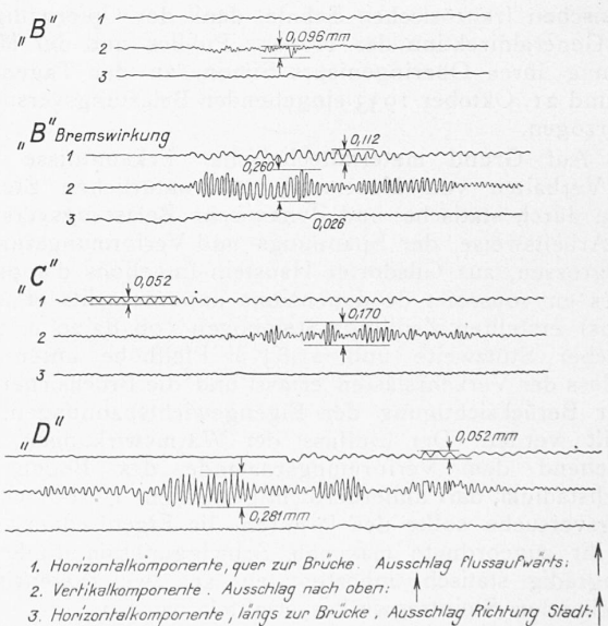
Abb. 5. Schwingungen des Bogens infolge Verkehrslast, gemessen mit dem Seismograph Trüb, Täuber & Cie., System de Quervain-Piccard.
