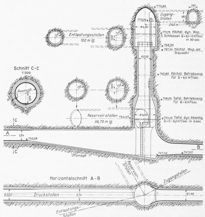
Abb. 17. Druckstollen (Schnitt C-C) 1 : 200 und Wasserschloss 1 : 400.
