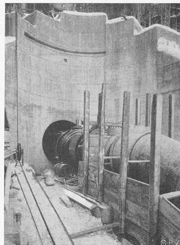
Abb. 19. Austritt der Druckleitung aus dem Rohrstoßen und der gebogenen Stützmauer.
