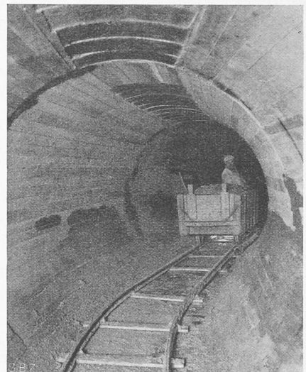
Abb. 16. Mit gehobelter und geölter Schalung betonierte Verkleidung bei WP III b.
