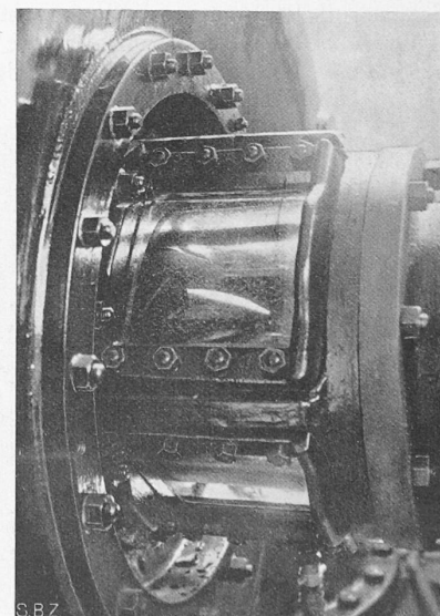
Abb. 15. Verglaste Schauöffnung am Laufradaustritt der Kavitationsturbine mit eingebautem Kaplan-Laufrad.
