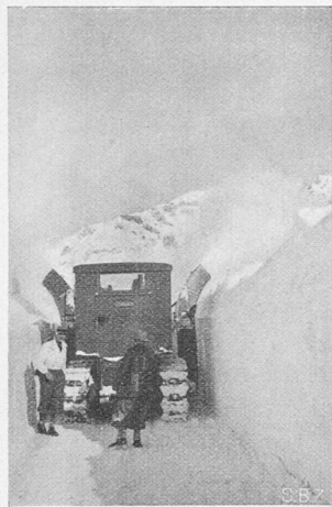
Abb. 10 und 11. Neue „Raco“-Cietrac-Schleuder am Arlberg: erster Schnitt.
