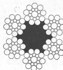
Seale- Konstruktion
