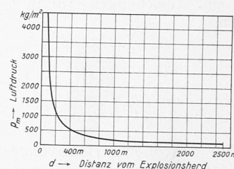
Abb. 1. Luftstoss einer 1000 kg Bombe (nach Schoszberger).
