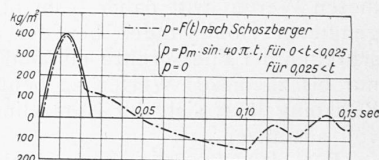
Abb. 2. Luftstoss p in Funktion der Zeit für d = 500 \text{ m} .
