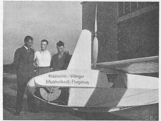
Abb. 1. Muskelkraft-Flugzeug Haessler-Villinger.
