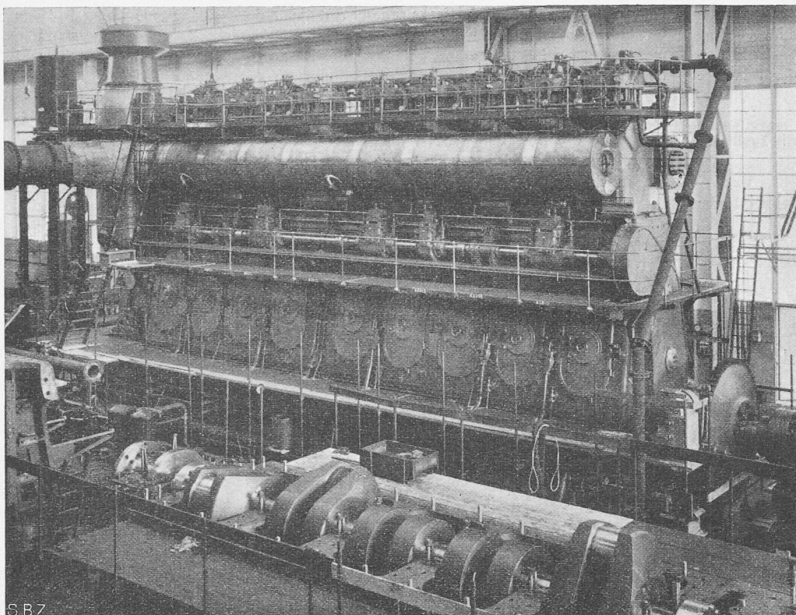
Abb. 1 (links). Einfachwirkender Sulzer-Zweitakt-Schiffsmotor, 6000 PS, 120 U/min. — Abb. 2 (rechts). Manövrierstand eines Zweitakt-Schiffsmotors, 6000 PS, 120 U/min. 1 Umsteuerhebel, 2 Maschinentelegraph, 3 Tachometer, 4 Hebel für „Anlassen“, „Betrieb“ und „Abstellen“, 5 Hebel mit Feineinstellung zum Regulieren der Brennstoffmenge
