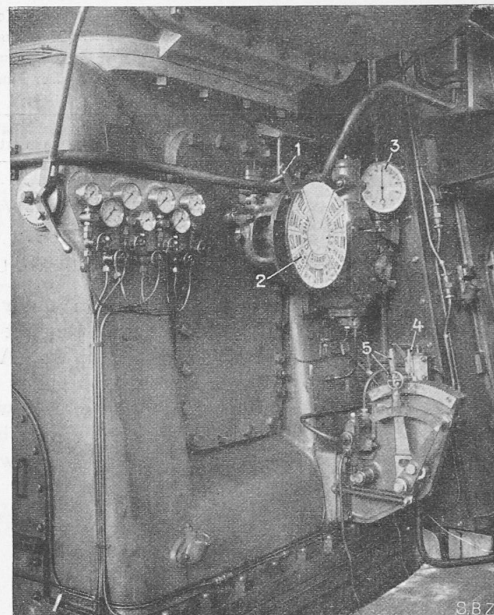
Abb. 1 (links). Einfachwirkender Sulzer-Zweitakt-Schiffsmotor, 6000 PS, 120 U/min. — Abb. 2 (rechts). Manövrierstand eines Zweitakt-Schiffsmotors, 6000 PS, 120 U/min. 1 Umsteuerhebel, 2 Maschinentelegraph, 3 Tachometer, 4 Hebel für „Anlassen“, „Betrieb“ und „Abstellen“, 5 Hebel mit Feineinstellung zum Regulieren der Brennstoffmenge
