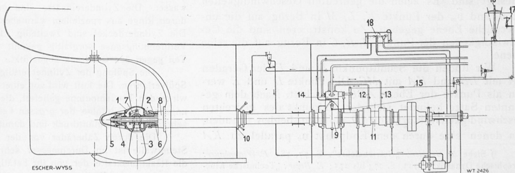
Abb. 4. Schematische Darstellung der Steuerung des Verstellpropellers beim Motorboot „Eitel“. (Legende im Text.)
