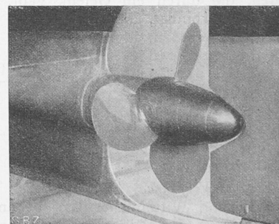
Abb. 2. Verstellpropeller.
