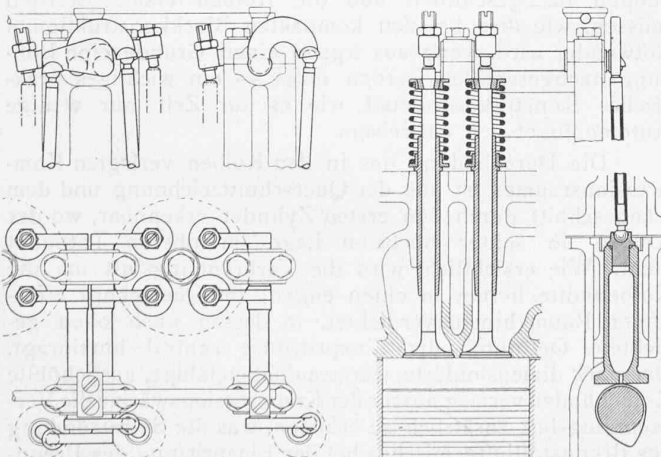
Abb. 6. Vierventil-Kipphebelsteuerung, 1:4.
