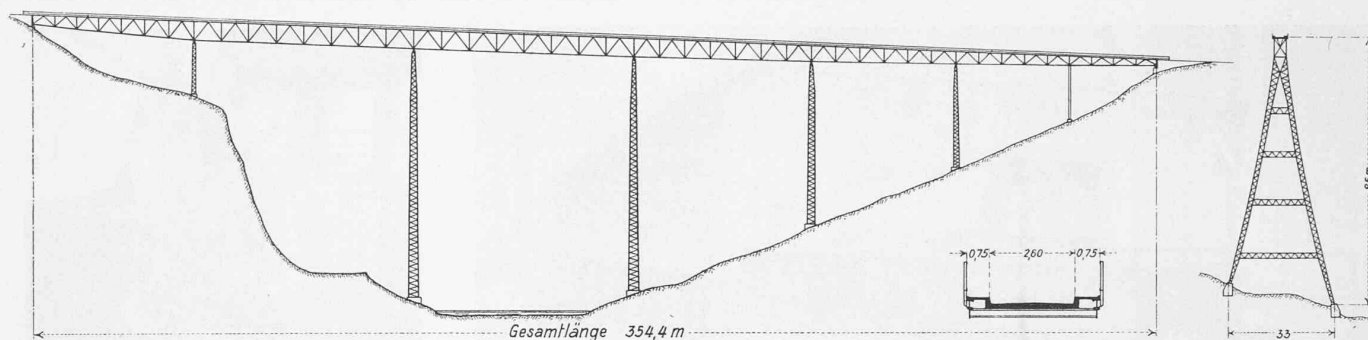
Eiserne Kleinverkehr-Strassenbrücke über die Sitter zwischen Hagen-Bruggen (links) und Stein, Appenzell (rechts). — Masstab 1 : 2200.
