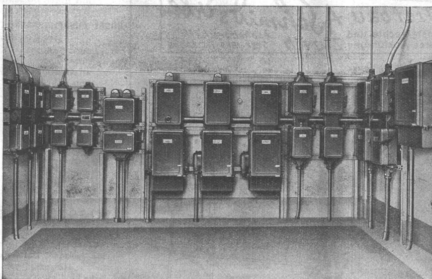
Gussgekapselte Niederspannungs-Verteilanlage
