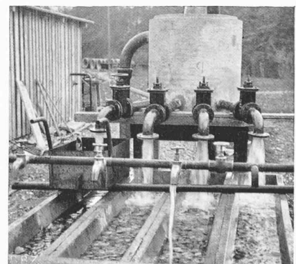
Abb. 3. Versuchsrinnen mit Beschiebung.
