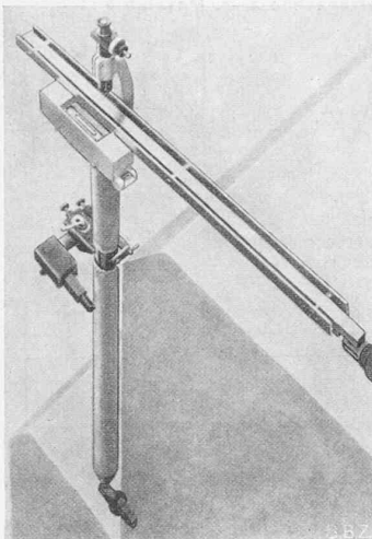
Abb. 8. Der Klinometerstab.
