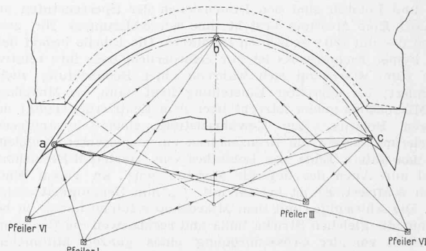
Abb. 7. Allgemeine Bogen- und Widerlagerbewegungen ermittelt auf Grund der kombinierten Winkel- und Längenmessungen. Sperrengrundriss 1 : 2500 mit den drei Beobachtungspfeilern a, b, c auf der Mauer und vier «Landpfeilern».
