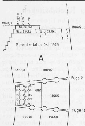
Abb. 5. Bewegungen eines Betonabschnittes unter dem Einfluss der Abbindevorgänge und der Temperaturänderungen:
