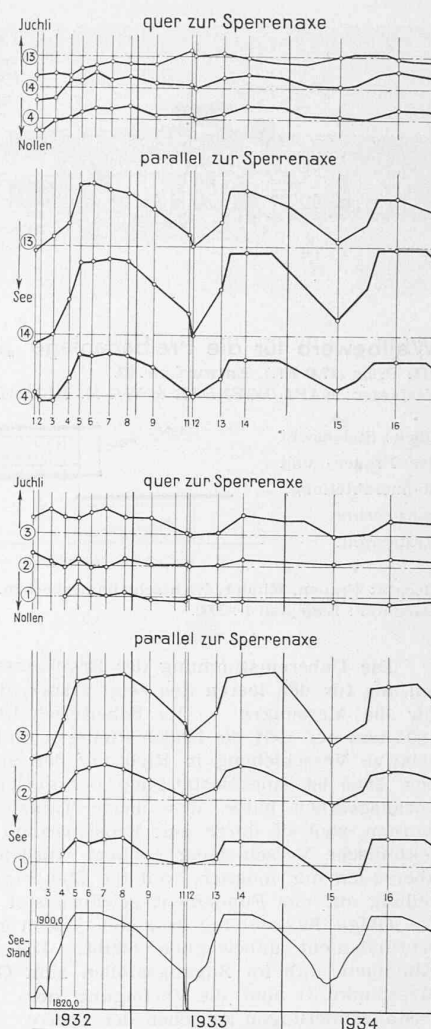
Abb. 12. Deformationsmessungen im Sperreninnern: relative Durchbiegungen, ermittelt mit dem Klinometerstab auf 2 m Höhe.
