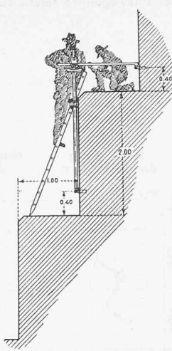
Abb. 9. Messung damit.
