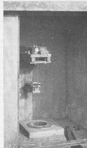
Abb. 10. Pendel-Aufhängung und Zentrierung. — Abb. 10 und 11 stammen nicht von der Grimsel, sondern von einer andern, ähnlichen Einrichtung an einer französischen Talsperre.
