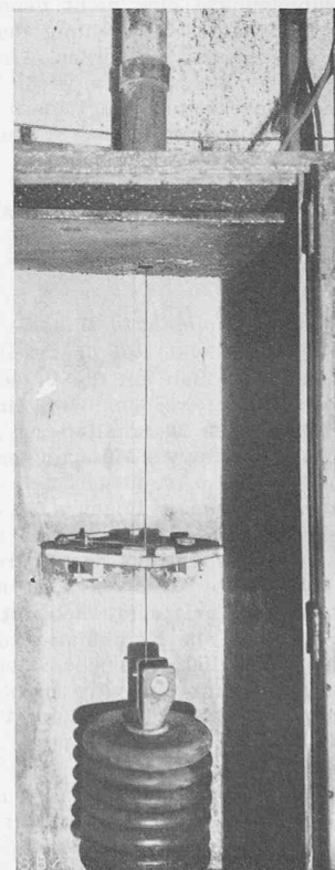
Abb. 11. Ablesetisch und Pendelgewicht.
