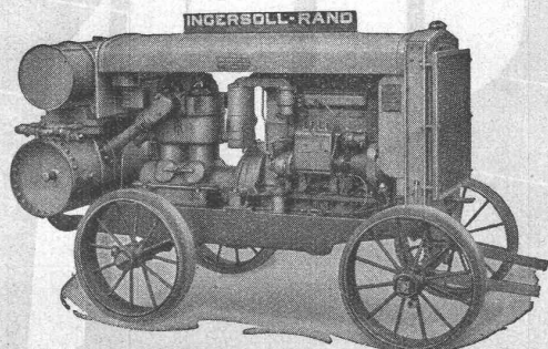
Rohölkompressor 20/26 PS.
