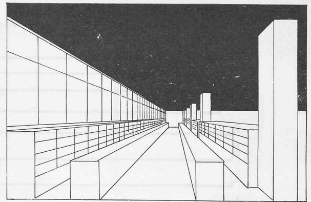
Abb. 2 und 3. Richtige Anordnung der Stützen bei ausgekragter Fassade. — Stützen zwischen den Regalen (Abb. 4, links) hindern die Uebersicht.
