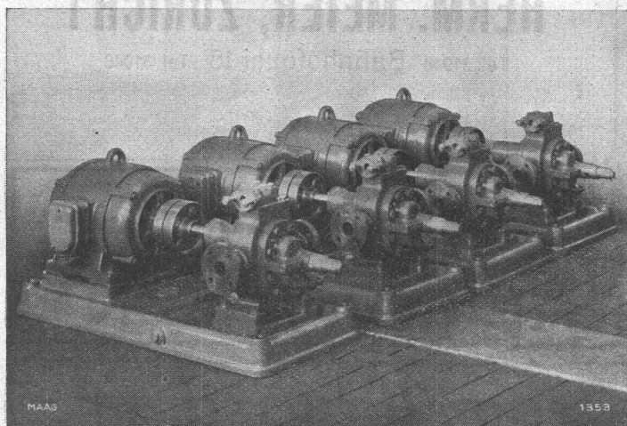
Maag-Zahnradpumpe Type M P 70 mit gehärteter und geschliffener Verzahnung, zur Förderung von Öl bei 250 °C; 3 at.
