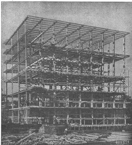
Stahlskelett des Kühlhhauses im Bahnhof Basel.
