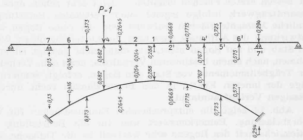
Abb. 8. Effektive Belastung des Stabes und des Bogens infolge P = 1 in 4.
