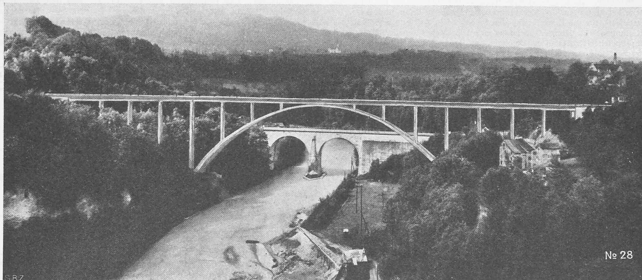
5. Rang (3000 Fr.), Entwurf Nr. 28. Ingenieurbureau BUSS A. G., Basel mit Arch. H. BAUR, Basel.
