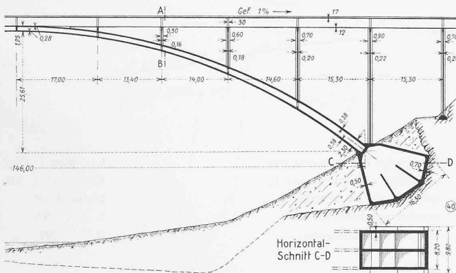
9. Rang (2250 Fr.), Entwurf Nr. 40. Eingespannter Eisenbetonbogen. Verfasser Ing. F. PFEIFFER, Zürich. Längsschnitt 1:1000.
