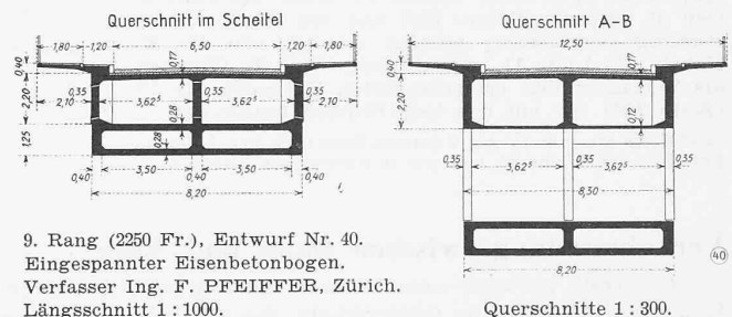
Querschnitte 1:300.
