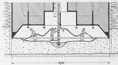
Abb. 14. Längsschnitt durch die Arbeitskammer während des Aushubbetriebes.
