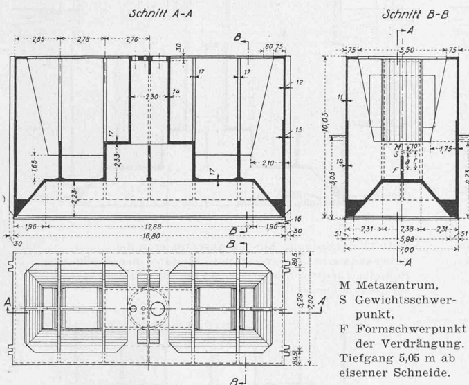
Abb. 8. Draufsicht und Schnitte der Eisenbetonsenkkasten 23 bis 38. Masstab 1 : 300.
