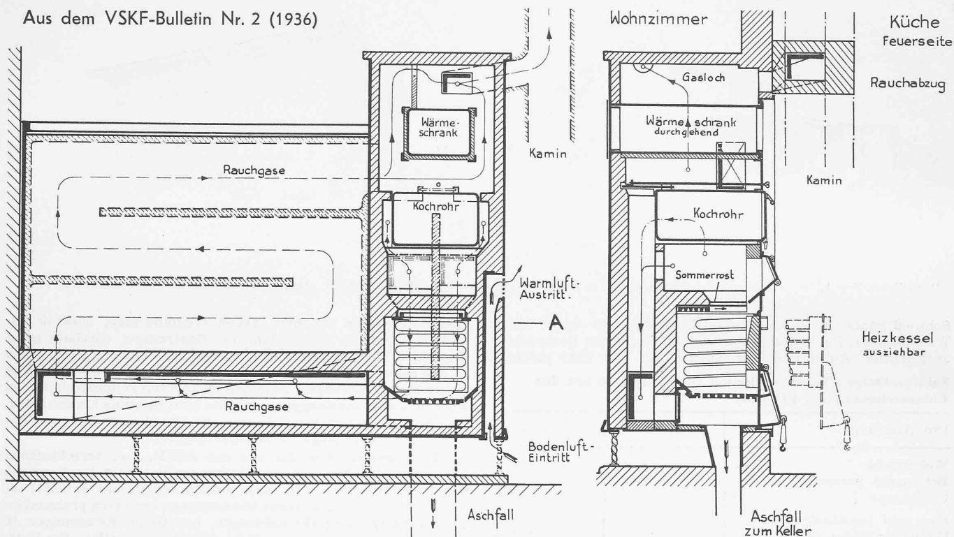
Kachelofen mit erwärmter Ofenbank (links), kombiniert mit Warmwasser-Heizung einiger Nebenräume (Etagenheizung).
