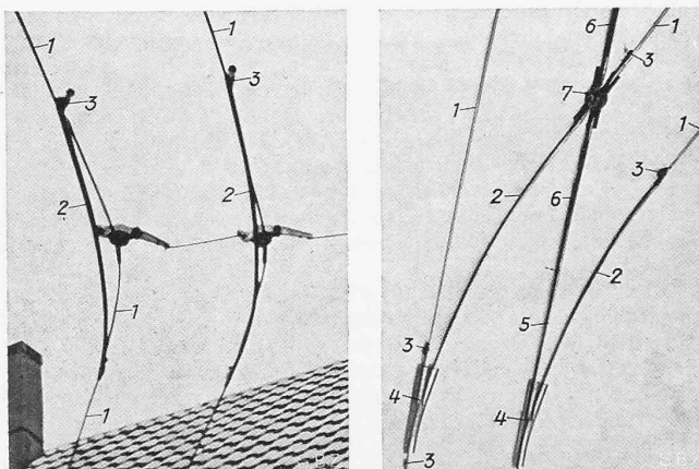
Abb. 13. Fahrleitungskurve und -Weiche mit stabilen Rohrbogenstücken Bauart Kummler & Matter (Aarau). 1 Fahrdracht; 2 Bogenstücke mit Uebergangsklemmen 3; 4 Weichen; 5 Verbindungsstück; 6 Stab-Isolatoren; 7 Kreuzungsstück.
