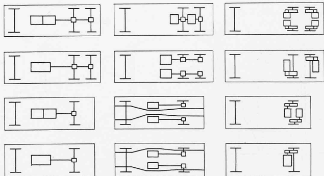
Abb. 6. Verschiedene Antriebsanordnungen für Trolleybusse.
