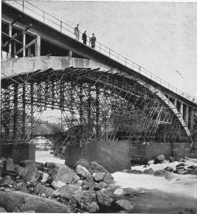
Abb. 5. Stahlrohr-Lehrgerüst einer Betonbrücke in Italien. — System «Innocenti». — Abb. 4. Deckengerüst in der «Basilica S. Paolo» in Rom.
