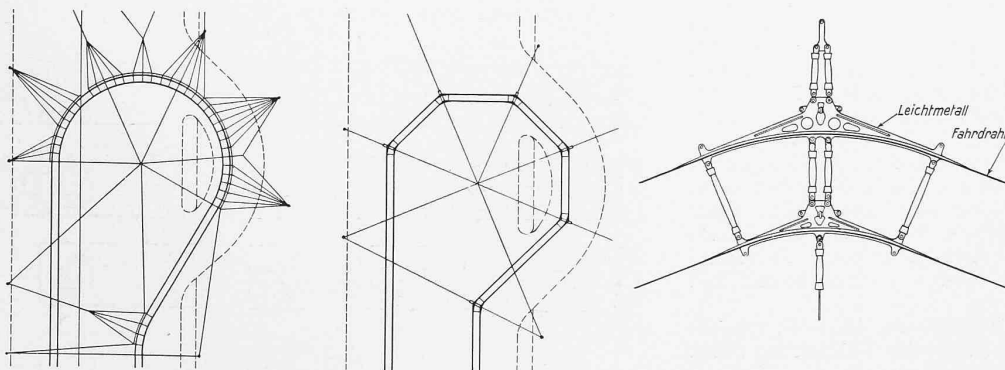
Abb. 11. Fahrleitungsschleifen: links in üblicher Bauart, rechts Bauart Westinghouse-Holden mit wenigen Stützpunkten und Leichtmetall-Kurvenstücken.
