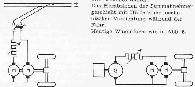
Als Trolleybus, Als Diesel- oder Benzinautobus laufend. Abb. 8. Antriebschema der Zweikraftwagen von Newark.
