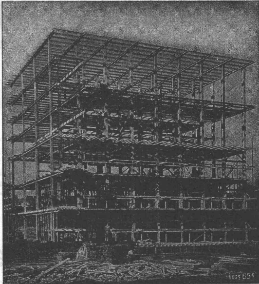
Stahlskelett des Kühllhauses im Bahnhof Basel.
