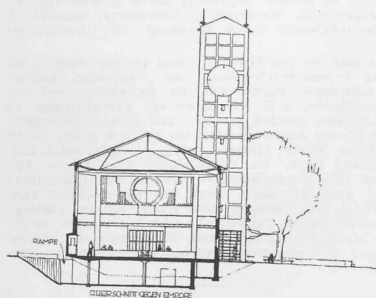
QUERSCHNITT GEGEN CHOR
