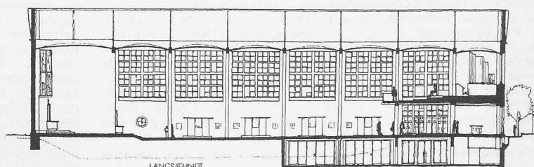
LÄNGSSCHNITT
