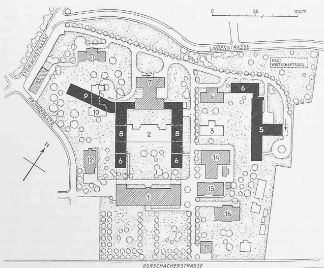
2. Preis, Entwurf Nr. 34. Lageplan 1: 4000 — Legende: 1 Medizin. Abt.; 2 (Haus 2) Bettenhaus Chirurg, Abt.; 3 (Haus 3); 4 Nasen- u. Ohrenklinik; 5 Frauenspital; 6 Personal; 7 Operationshaus; 8 Chirurgie; 9 Kinder- und Tuberkulosehaus; 10 Entbindungsanstalt; 11 Absonderungshaus; 12 Prosektur; 13 Werkstätten; 14 Wäscherei und Kesselhaus; 15 Kochküche; 16 Augenklinik; 17 Verwaltung.
