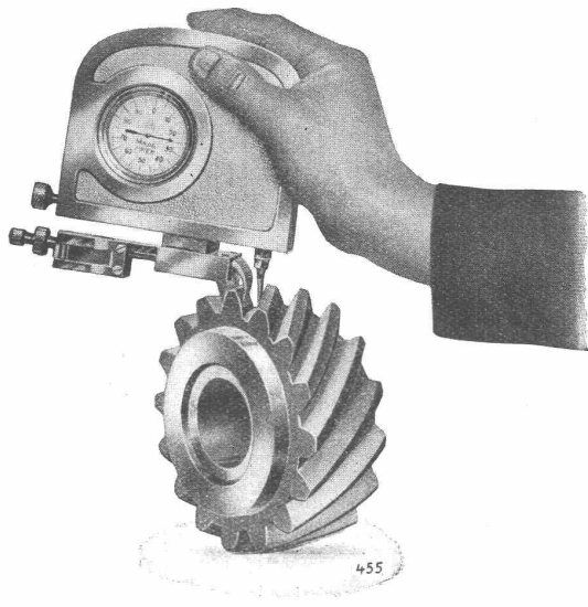
Maag-Zahnradprüfapparat TME zur Kontrolle der Zahnprofile und Normalteilungen.
