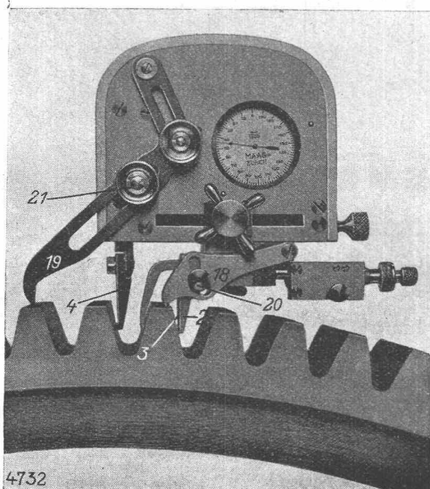
Maag-Teilungsmessinstrument zur vergleichenden Messung von Kreisteilungen, Type TMA.
