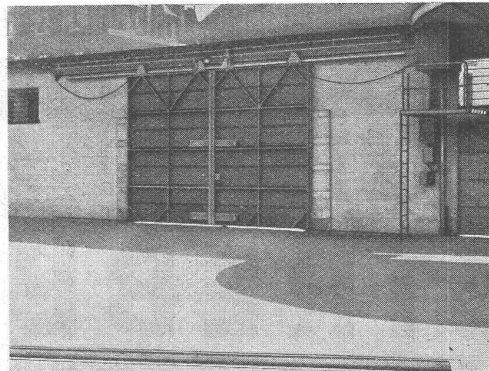
Schiebetor mit elektr. Antrieb und Kontaktleiste zum autom. Oeffnen des Tores
