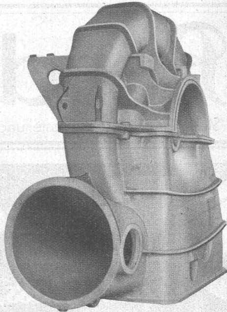
(Gebläsegehäuse) Dimensionen: Höhe 2600 mm, Länge 2500 mm, Breite 1200 mm, Gewicht ca. 1325 kg.
