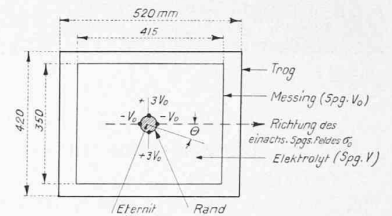
Abb. 2. Anordnung zum Lochversuch. Gesteuerte Punkte 36, d. h. alle 10°.
