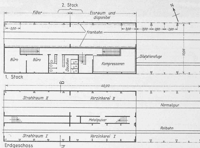
Abb. 10. Metallspritzwerk. Grundrisse 1:400
