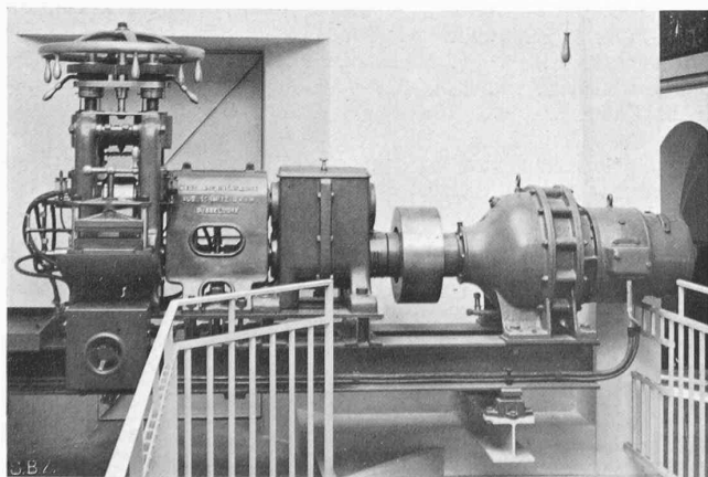
Abb. 3. Kleines Walzwerk für Rundmaterialien und Bänder
