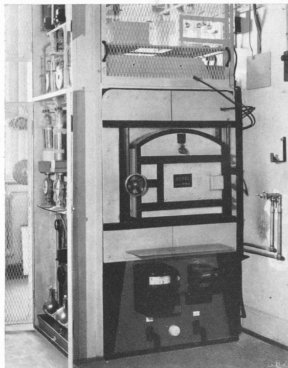
Abb. 2. Auskühllofen der Firma Borel (Peseux)
