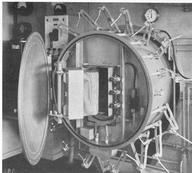
Abb. 4. Muffelofen für max. 1450°C der Firma Brown, Boveri (Baden)
