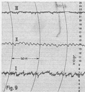
Dr. Frenzel-Diagramme: Abb. 10 (Fig. 8) A Flachsgarn, B Baumwollgarn, \frac{3}{4}\% Gesamtdehnung. - Abb. 11 (Fig. 9) I Wollstreichgarn, II Baumwollgarn (Wellen wegen Ringbankspielen), III Viscosegarn, je bei 70\% der Bruchdehnung (Viscose als Kunstprodukt sehr gleichmässig). - Abb. 12 (Fig. 10) Schlechtes Baumwollgarn, 4\frac{1}{2}\% Gesamtdehnung (1 bis 4 Fadenbrüche)
