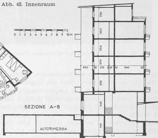
Abb. 43. Innenraum
