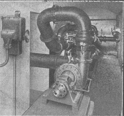
Niederdruck-Zentrifugalpumpe 160 P.S.
