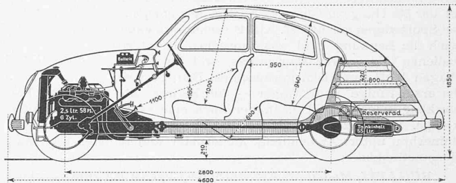
Abb. 10. Adler, Modell 2500, mit guter Raumaussnutzung. — 1:50
