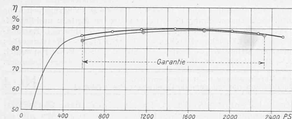
Abb. 4. Ergebnisse der Leistungsversuche an der Bannalp-Turbine 1
