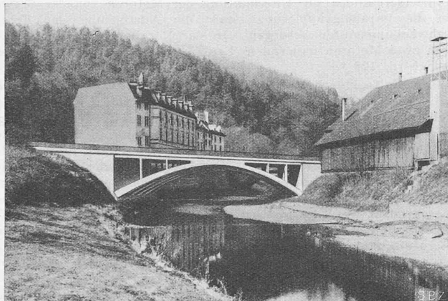
III. Preis (1100 Fr.), Entwurf Nr. 2. — Verfasser: Ing. CH. CHOPARD (Zürich), Mitarbeiter Ing. MAX MEYER (Zürich) mit STRAULI & RÜEGGER, Architekten (Winterthur)
