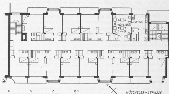
Abb. 2. Grundriss vom ersten Stock. — Masstab 1 : 400
