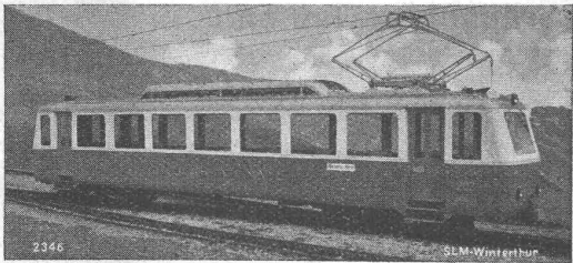
Elektr. Zahnrad-Triebwagen für die Glion-Rochers de Naye-Bahn
