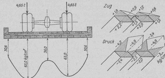
Abb. 17. Fahrbahn
