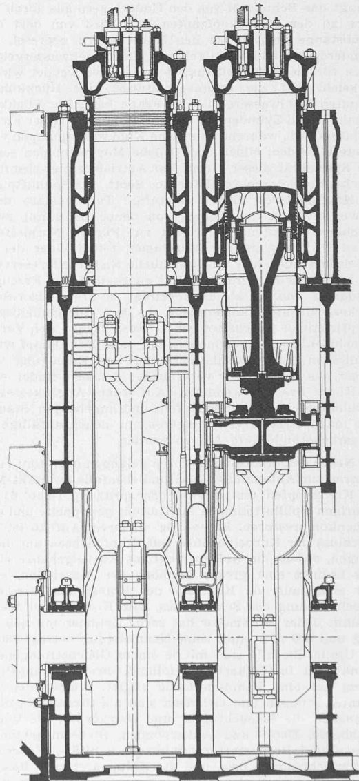
Abb. 2. Längsschnitt durch zwei Zylinder einer Hauptmaschine
