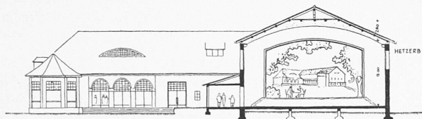
ALTBAU OST-ANSICHT
