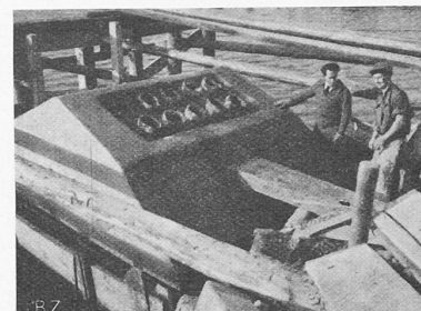
Abb. 51 und 52. Streben-Fundament des Schwebebahn-Turmes auf dem rechten Ufer
